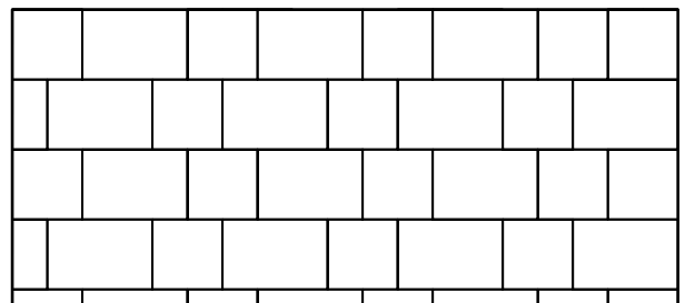
Muster Nr. DEC 2L 142 , Berechnungsschlüssel für 1 m 2 :
