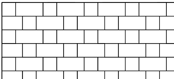
Muster Nr. DEC 2L 141 , Berechnungsschlüssel für 1 m 2 :
