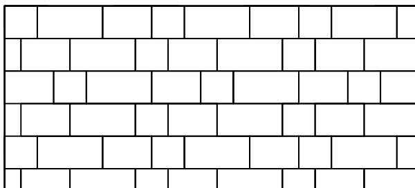
Muster Nr. DEC 3L 163 , Berechnungsschlüssel für 1 m²:
