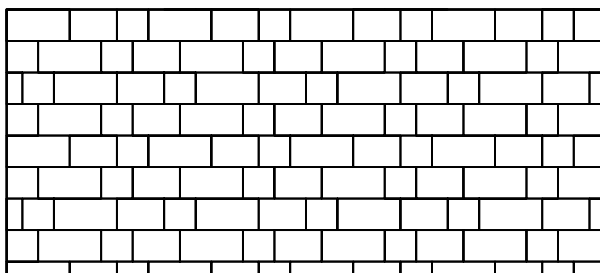
Muster Nr. DEC 3L 165 , Berechnungsschlüssel für 1 m²:
