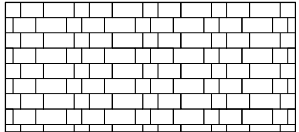
Muster Nr. DEC 3L 160 , Berechnungsschlüssel für 1 m²:
