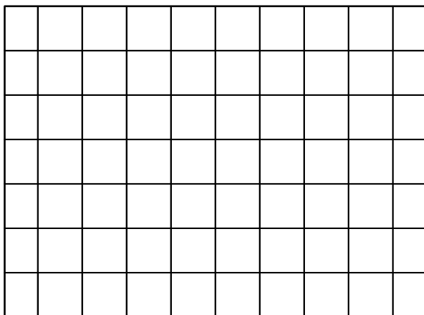
Muster Nr. GPL 1391 , Berechnungsschlüssel für 1 m 2 : ca. 6,19 Stk Gartenplatte 39,7x39,7
