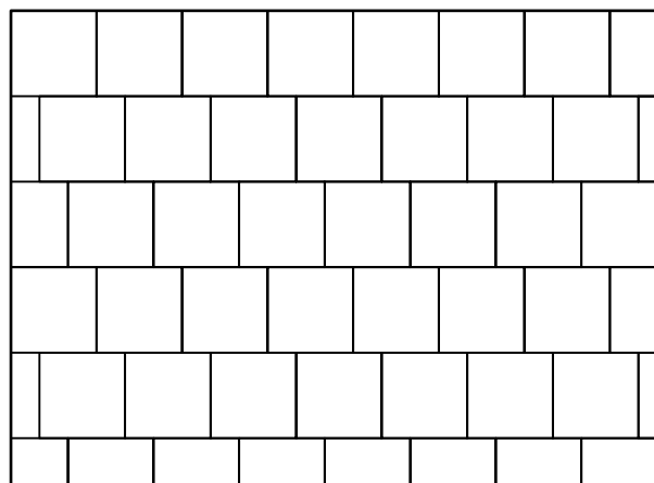
Muster Nr. GPL 1493 , Berechnungsschlüssel für 1 m 2 : ca. 3,97 Stk Gartenplatte 49,7x49,7
