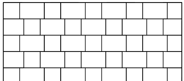
Muster Nr. TEG 2L 545 , Berechnungsschlüssel für 1 m²: ca. 3,19 Stk Tegula16 Platte 34,6x34,6 ca. 3,19 Stk Tegula16 Großplatte 52,2x34,6
