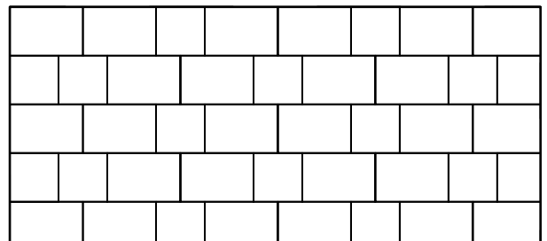
Muster Nr. TEG 2L 543 , Berechnungsschlüssel für 1 m²: ca. 2,00 Stk Tegula16 Platte 34,6x34,6 ca. 3,99 Stk Tegula16 Großplatte 52,2x34,6
