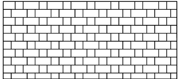
Muster Nr. TEG 2L 541 , Berechnungsschlüssel für 1 m²: ca. 10,64 Stk Tegula16 Quadratstein 16,9x16,9 ca. 10,64 Stk Tegula16 Halbplatte 34,6x16,9
