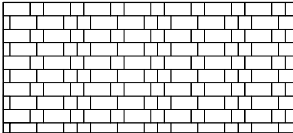
Muster Nr. TEG 2L 540 , Berechnungsschlüssel für 1 m²: ca. 10,64 Stk Tegula16 Quadratstein 16,9x16,9 ca. 10,64 Stk Tegula16 Halbplatte 34,6x16,9
