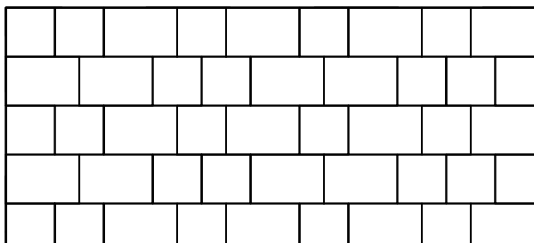
Muster Nr. TEG 2L 544 , Berechnungsschlüssel für 1 m²: ca. 3,19 Stk Tegula16 Platte 34,6x34,6 ca. 3,19 Stk Tegula16 Großplatte 52,2x34,6
