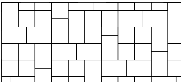
Muster Nr. TEG 2F 607 , Berechnungsschlüssel für 1 m 2 :
