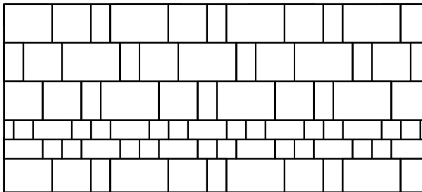
Muster Nr. TEG 2BL 589 , Berechnungsschlüssel für 1 m 2 :
