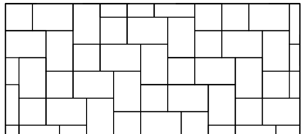
Muster Nr. TEG 2F 608 , Berechnungsschlüssel für 1 m 2 :
