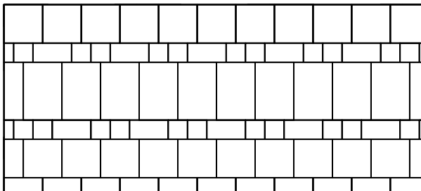
Muster Nr. TEG 3BL 596 , Berechnungsschlüssel für 1 m 2 :
