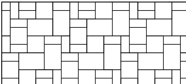
Muster Nr. TEG 3F 630 , Berechnungsschlüssel für 1 m 2 :
