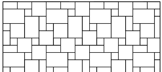
Muster Nr. TEG 4F 640 , Berechnungsschlüssel für 1 m 2 :
