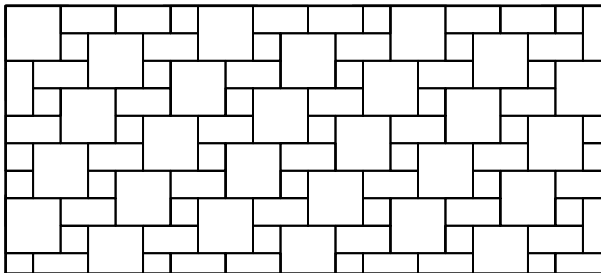
Muster Nr. TEG 3F 626 , Berechnungsschlüssel für 1 m 2 :
