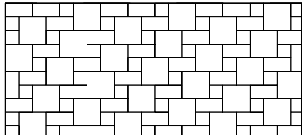
Muster Nr. TEN 3F 426 , Berechnungsschlüssel für 1 m²:
