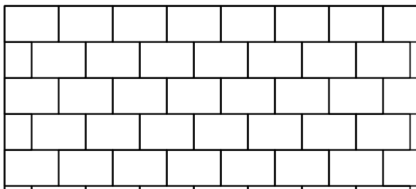
Muster Nr. TEK 1L 705 , Berechnungsschlüssel für 1 m²: ca. 6,12 Stk Tegula K&K Binderplatte 48,7x32,2
