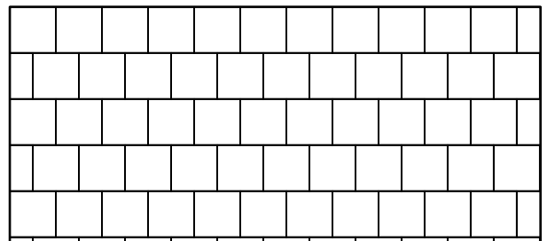
Muster Nr. TEK 1L 704 , Berechnungsschlüssel für 1 m²: ca. 9,18 Stk Tegula K&K Platte 32,2x32,2
