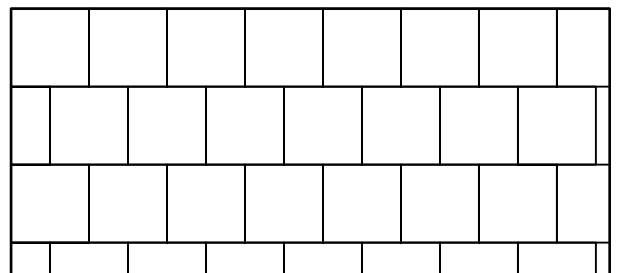
Muster Nr. TEK 1L 708 , Berechnungsschlüssel für 1 m²: ca. 4,08 Stk Tegula K&K Großplatte 48,7x48,7
