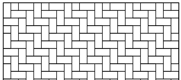
Muster Nr. TEK FG 721 , Berechnungsschlüssel für 1 m²: ca. 18,37 Stk Tegula K&K Halbplatte 32,2x15,7
