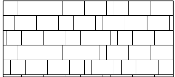
Muster Nr. TEK 3L 771 , Berechnungsschlüssel für 1 m 2 :
