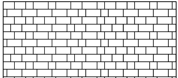
Muster Nr. TEK 3L 773 , Berechnungsschlüssel für 1 m 2 :
