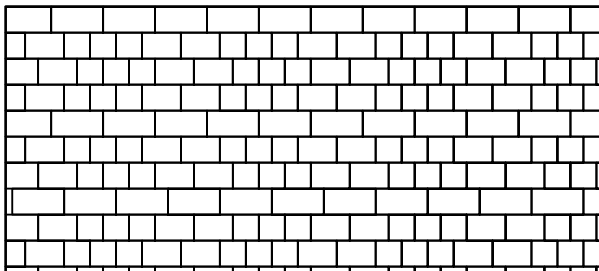
Muster Nr. TEK 3L 774 , Berechnungsschlüssel für 1 m 2 :
